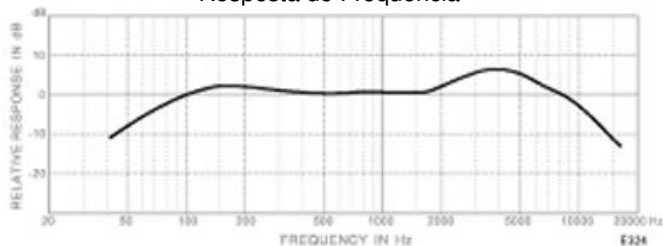
Resposta de Freqüência
