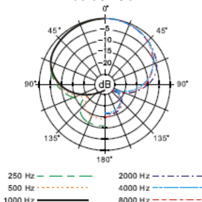
Padrão Polar
