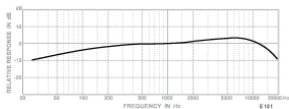
Resposta de Frequência
