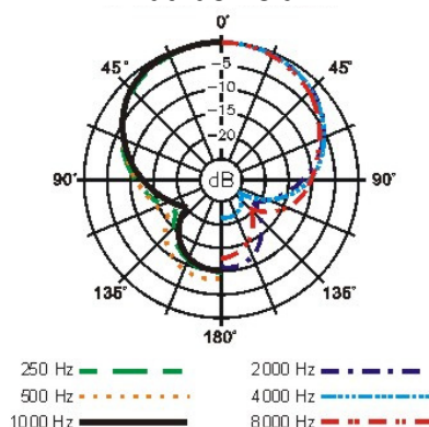
Padrão Polar
