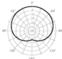
Padrão Polar
